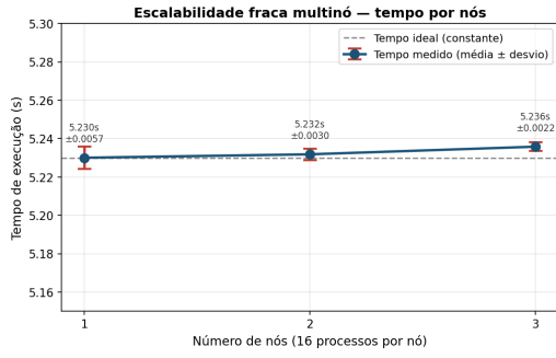
Figura 10. Escalabilidade fraca multinó: tempo de execução em função do número de nós, com barras de erro (desvio padrão de 5 execuções). Fonte: elaborado pelos autores (2026).
