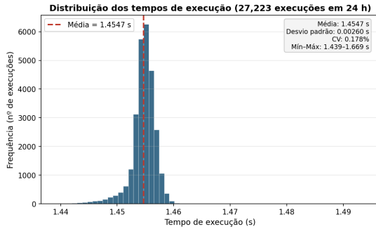
Figura 12. Distribuição dos tempos de execução das 27.223 execuções bem-sucedidas em 24 horas. Fonte: elaborado pelos autores (2026).
