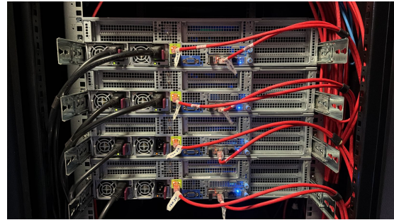
Figura 2. Vista traseira: cabeamento de rede, alimentação redundante e interfaces de gerenciamento. Fonte: elaborado pelos autores (2026).
