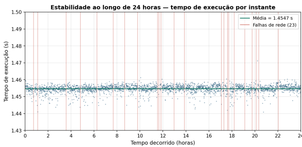
Figura 13. Tempo de execução ao longo das 24 horas. As linhas verticais indicam as 23 falhas de comunicação de rede. Fonte: elaborado pelos autores (2026).
