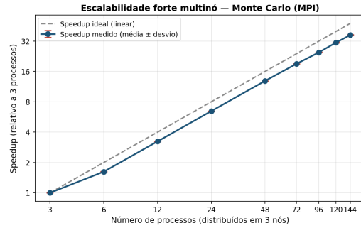
Figura 9. Speedup em escalabilidade forte multinó (3 a 144 processos em 3 nós), com barras de erro (desvio padrão de 10 execuções). Fonte: elaborado pelos autores (2026).
