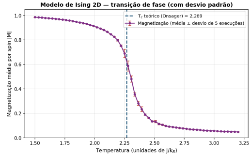
Figura 11. Modelo de Ising 2D: magnetização média por spin em função da temperatura, com barras de erro (desvio padrão de 5 execuções). A linha tracejada indica a temperatura crítica teórica de Onsager. Fonte: elaborado pelos autores (2026).
